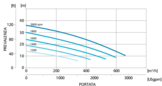
PAS 300MF 401
