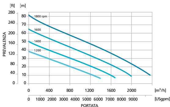
PAS 300HF 440
